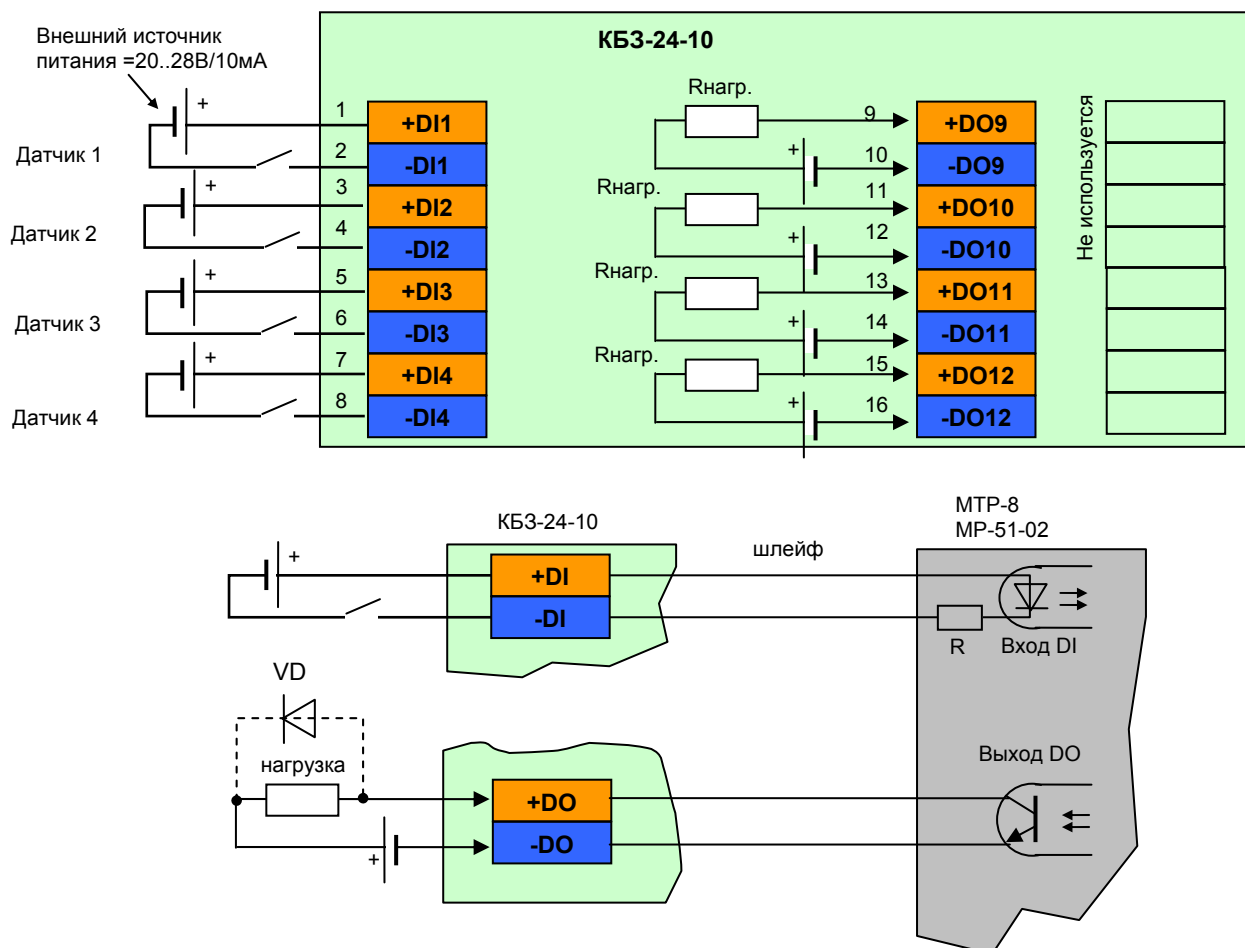
Рисунок Б.3.2.2 - Подключение сигналов модуля расширения МР-51-02 с помощью клеммно-блочного соединителя КБ3-24-10
