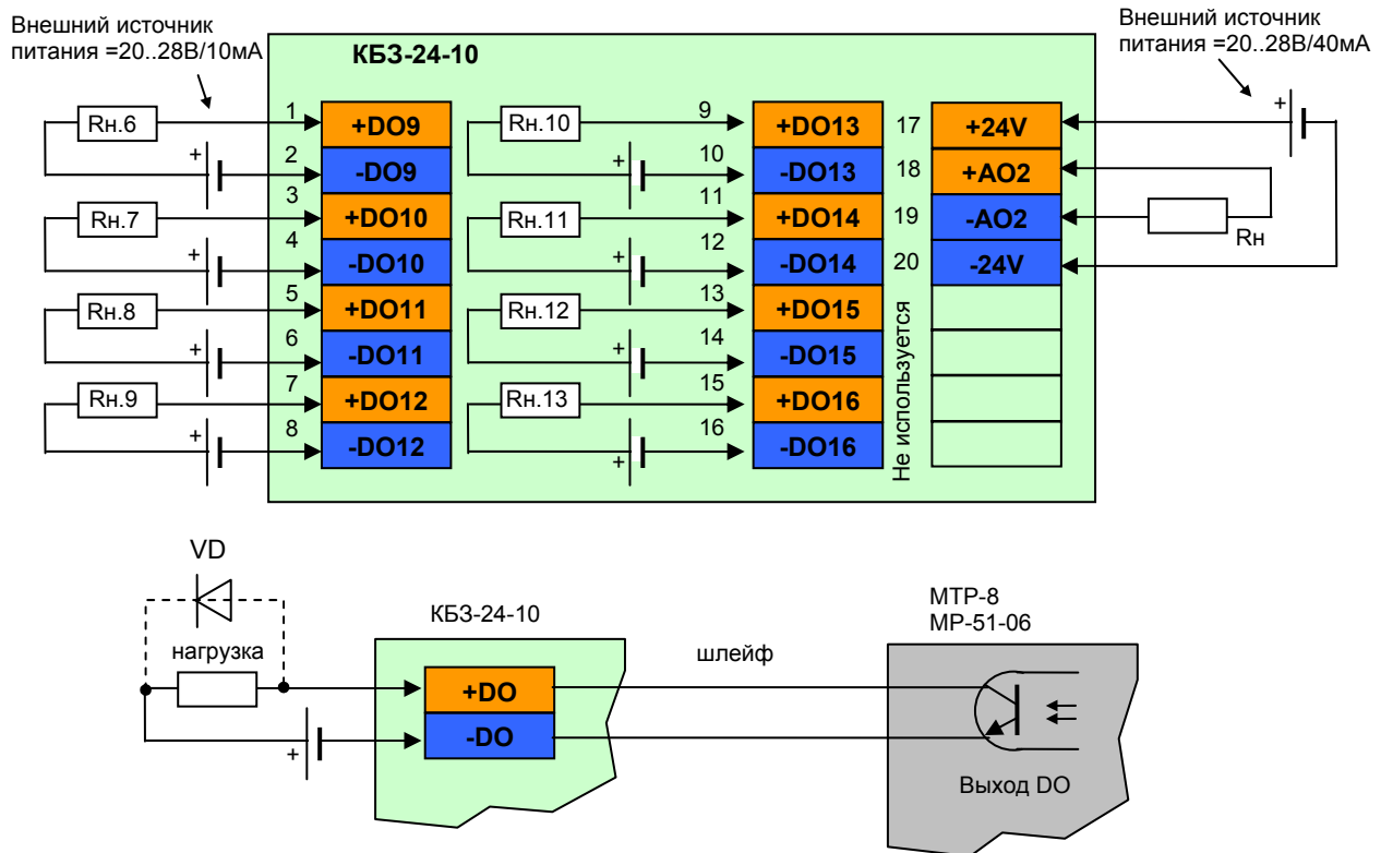
Рисунок Б.3.2.8 - Подключение сигналов модуля расширения МР-51-06 с помощью клеммно-блочного соединителя KB3-24-10
