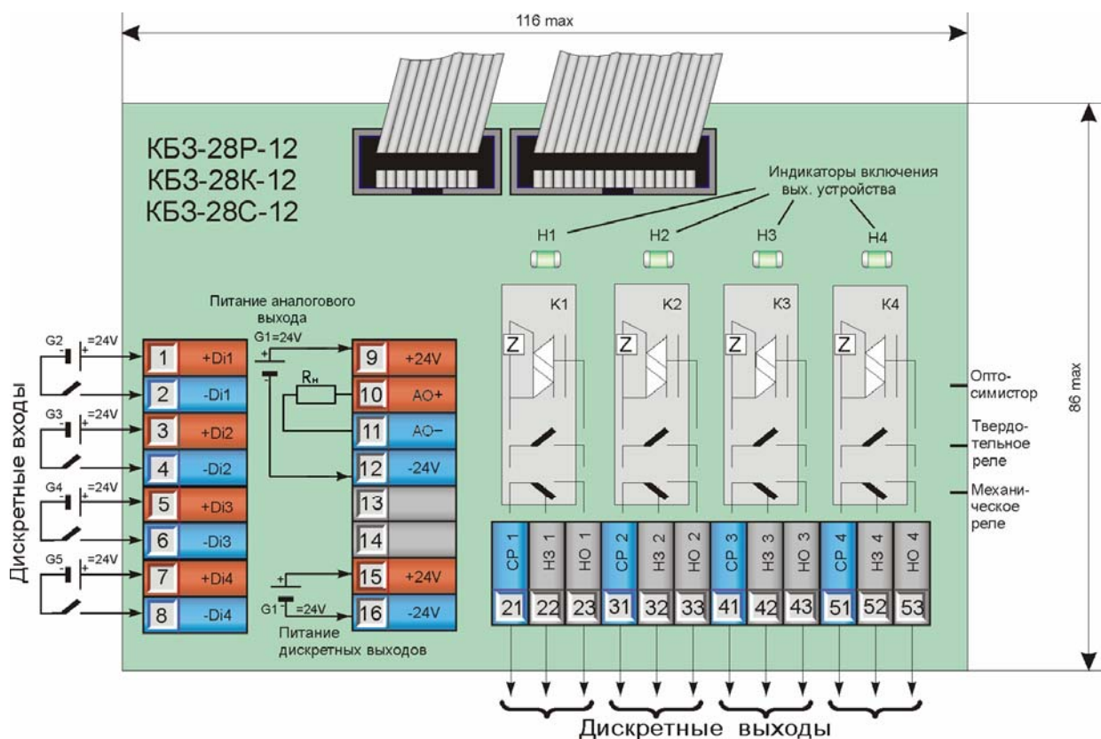
Рисунок Б.3.2.7 - Подключение сигналов модуля расширения МР-51-05 с помощью клеммно-блочного соединителя КБЗ-28Р-12, КБЗ-28С-12, КБЗ-28К-12
