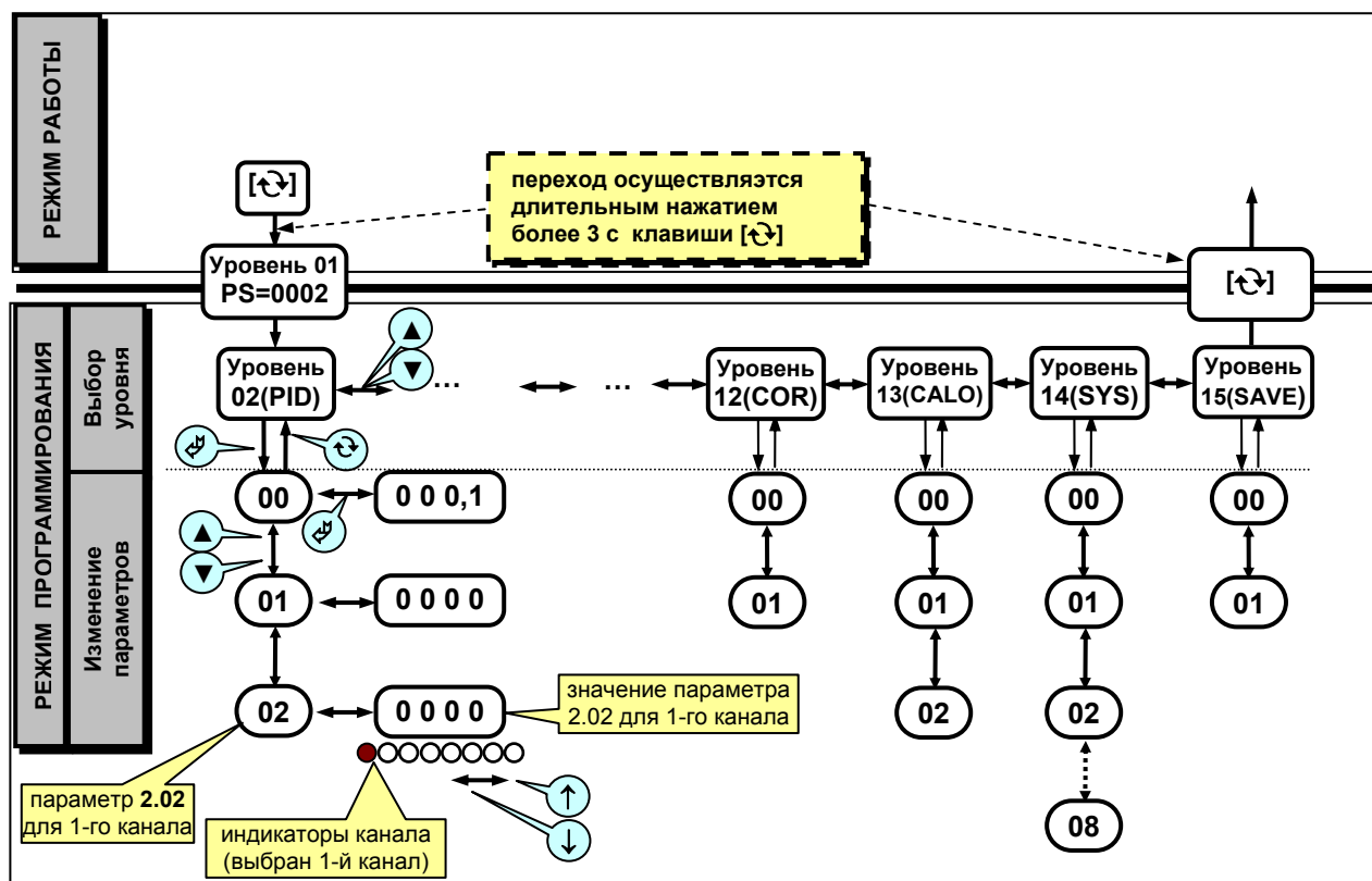
Рисунок 6.2 - Диаграмма уровней конфигурации и настроек
