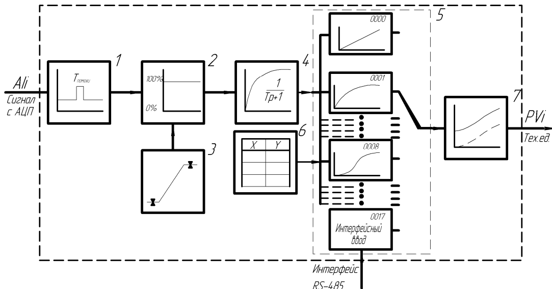
Рисунок 5.3 – Блок-схема обработки аналогового входа
