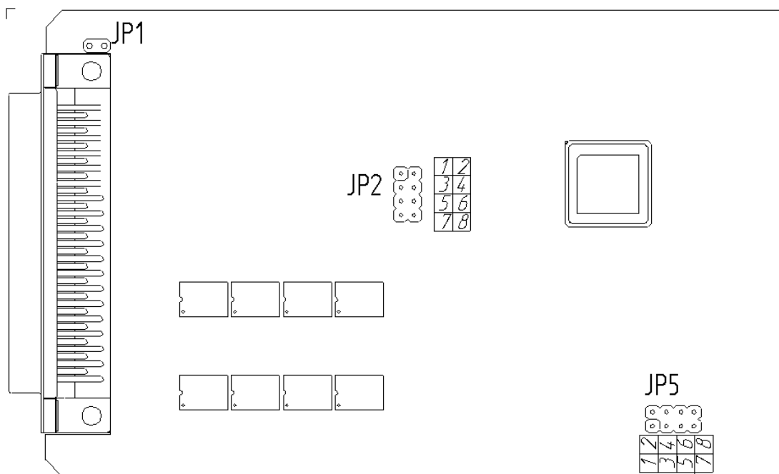
Рисунок 10.1 – Положение переключателей на плате процессора
