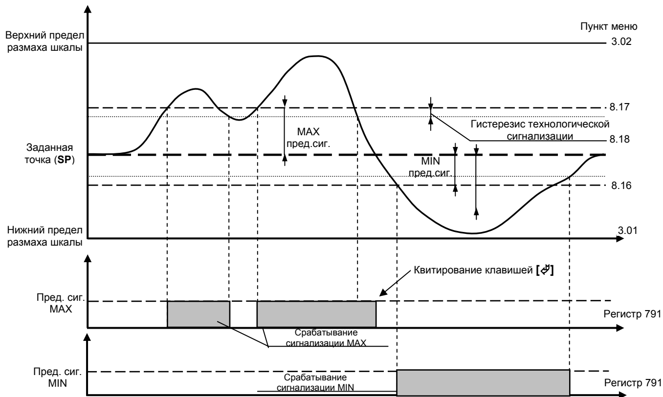
Рисунок 5.10 - График срабатывания девиационной предупредительной сигнализации с запоминанием или без п.8.15=0001, 0003
