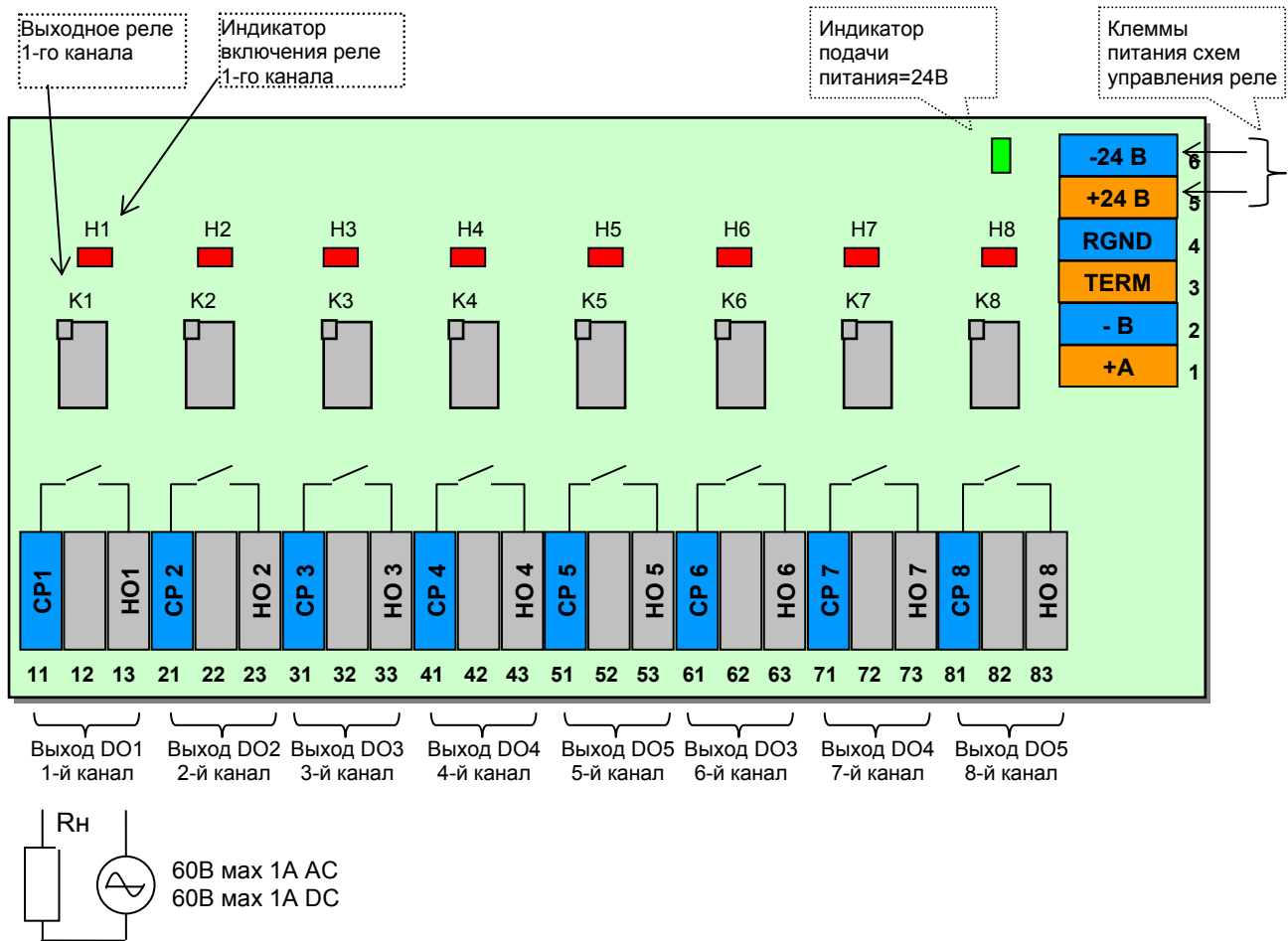
Рисунок Б.3.1.4-расположение сигналов и габаритные размеры клеммно-блочного соединителя КБ3-30К-11
