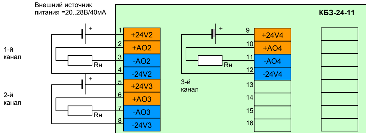
Рисунок Б.3.2.10 - Подключение сигналов модуля расширения МР-51-07 с помощью клеммно-блочного соединителя KB3-24-11
