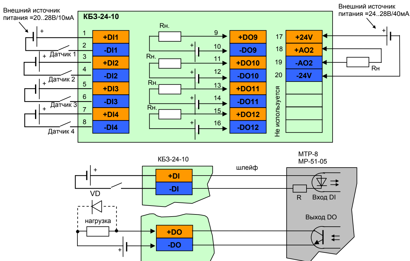
Рисунок Б.3.2.6 - Подключение сигналов модуля расширения МР-51-05 с помощью клеммно-блочного соединителя KB3-24-10
