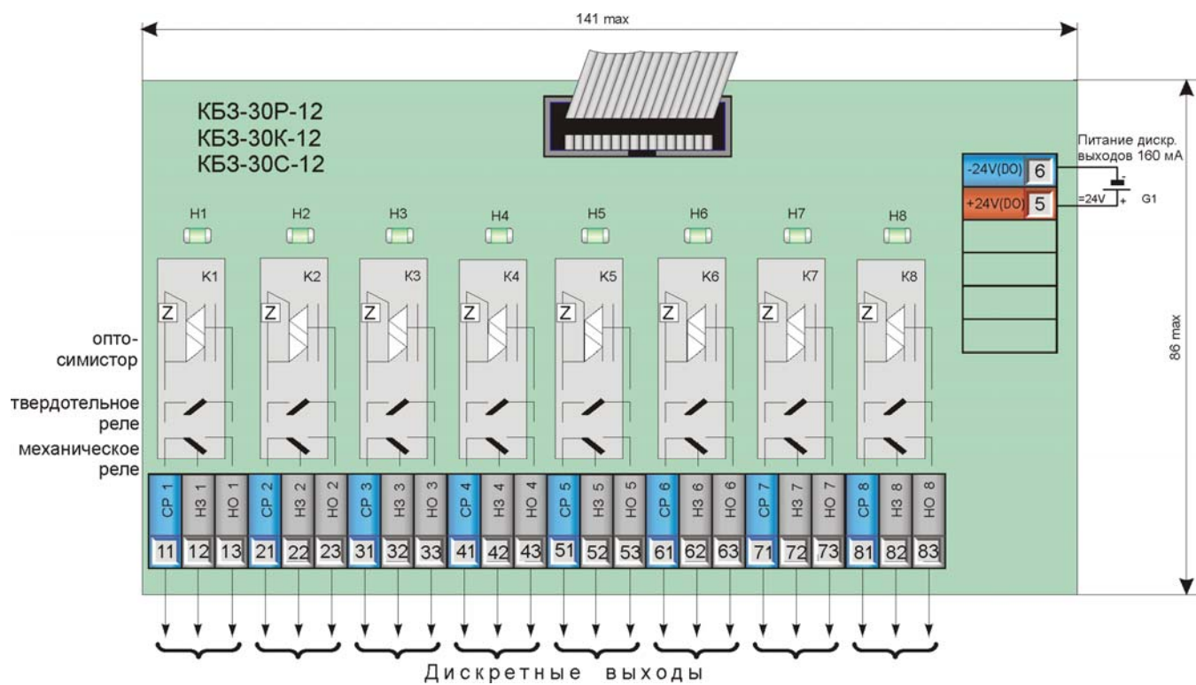
Рисунок Б.3.2.9 - Подключение сигналов модуля расширения МР-51-06 с помощью клеммно-блочного соединителя КБЗ-30Р-12, КБЗ-30К-12, КБЗ-30С-12
