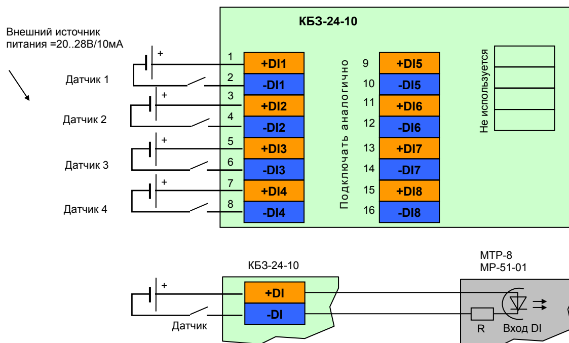
Рисунок Б.3.2.1 - Подключение сигналов модуля расширения МР-51-01 с помощью клеммно-блочного соединителя КБЗ-24-10
