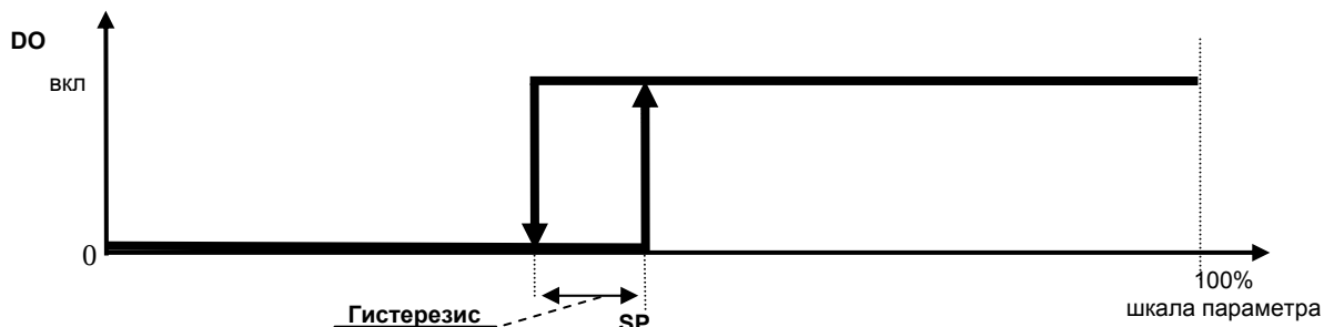
Рисунок 5.7 – Пример работы выходного устройства по логике прямого 2-х позиционного управления п.8.00=0001, п.8.02=0001
