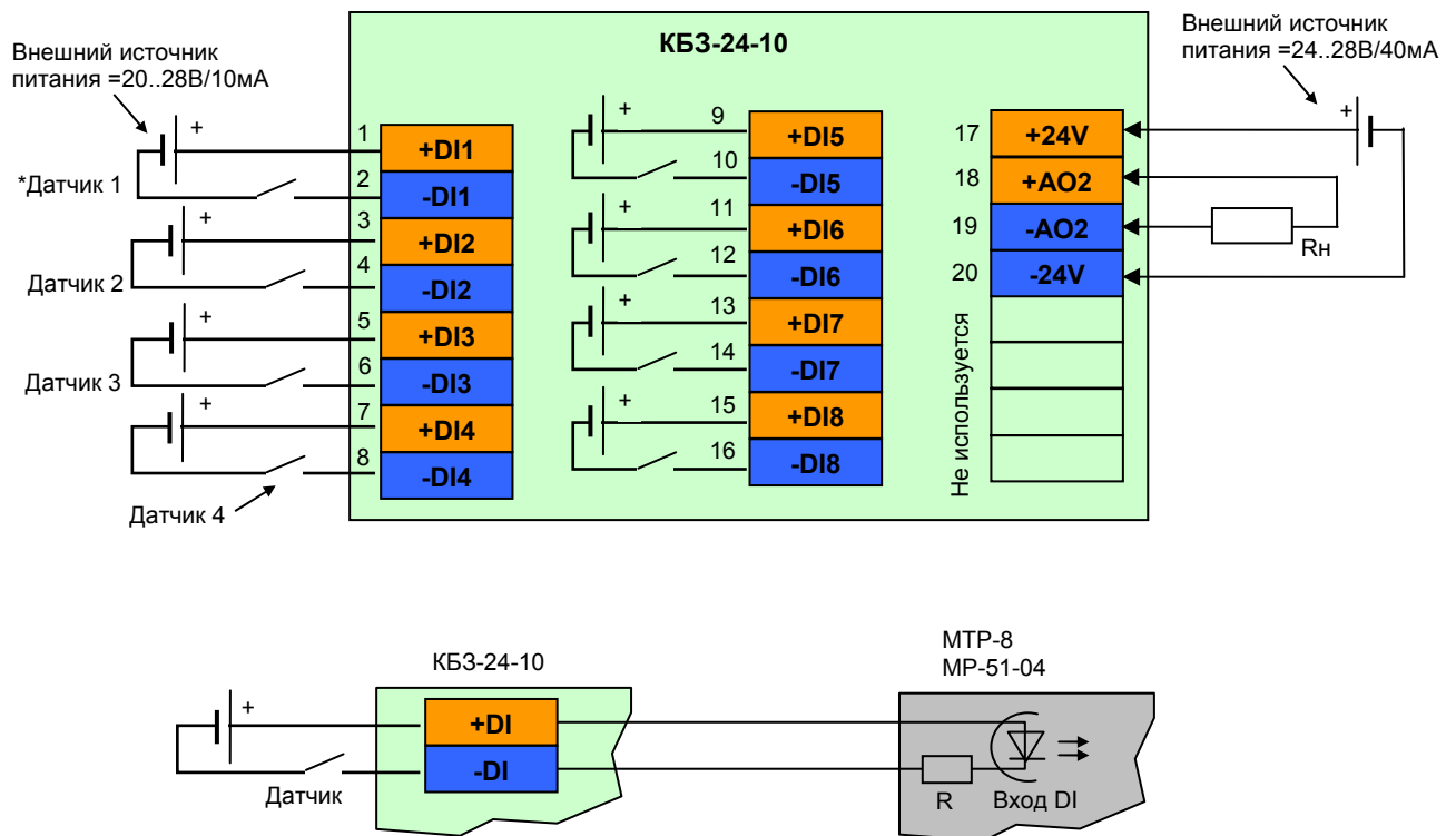
Рисунок Б.3.2.5 - Подключение сигналов модуля расширения МР-51-04 с помощью клеммно-блочного соединителя КБ3-24-10
