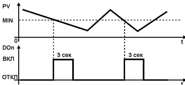
Рисунок 5.8 – График работы дискретного выхода при импульсном типе выходного сигнала
