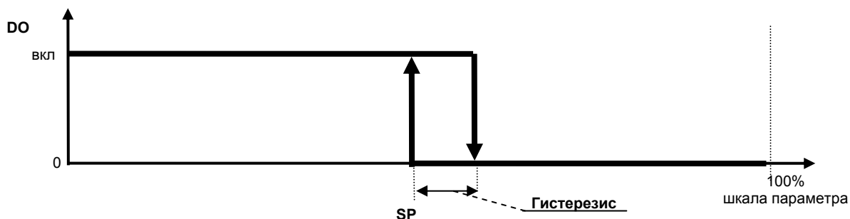
Рисунок 5.6 – Пример работы выходного устройства по логике обратного 2-х позиционного управления п.8.00=0001, п.8.02=0000
