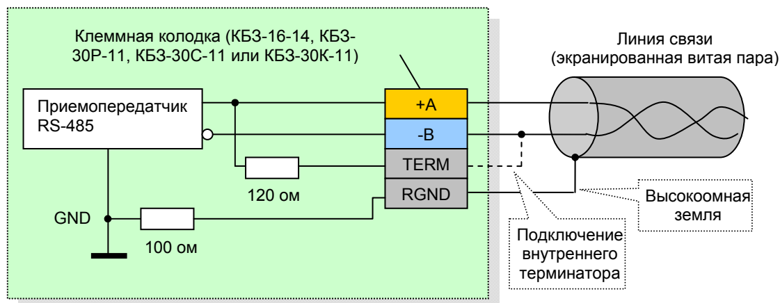
Рисунок Б.4.1 - Рекомендуемая схема подключения интерфейса RS-485
