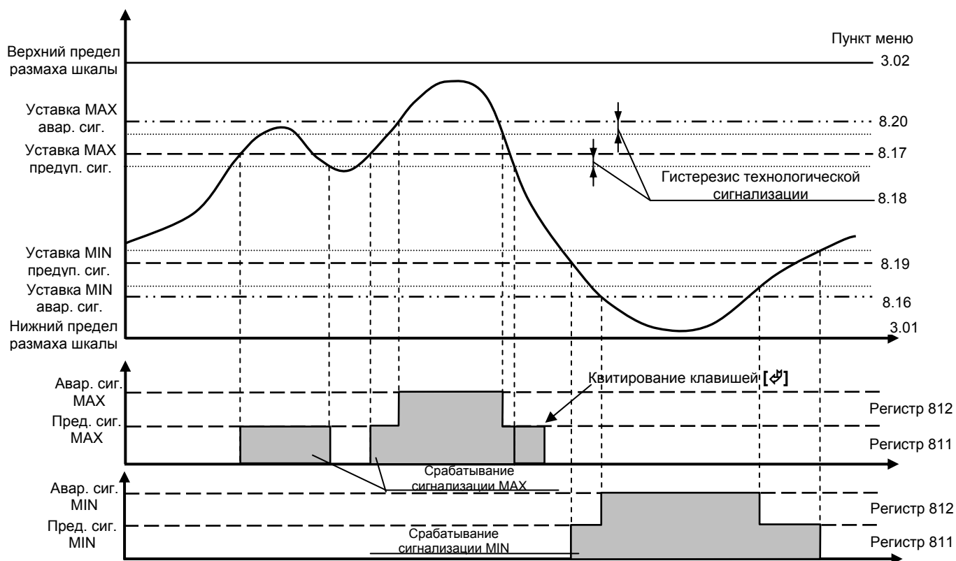
Рисунок 5.9 - График срабатывания абсолютной сигнализации с запоминанием или без п.8.15=0000, 0002
