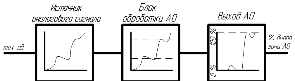
Рисунок 5.5 – Работа блока аналогового вывода в режиме ретрансмиссии
